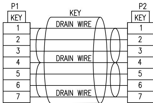
WIRING TABLE
